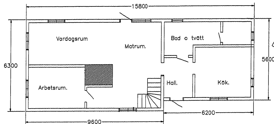
Plan befintlig nedre våning.
