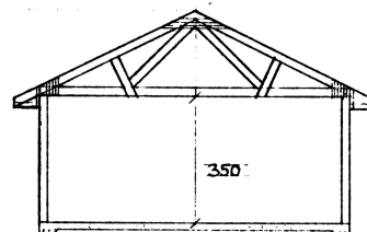
GARAGESEKTION
